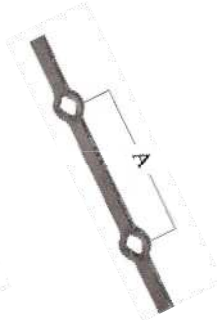
08.013 H 2000 mm A 140 mm □ 14x14 mm 14 otworów ◇ 14mm 3,080 kg
