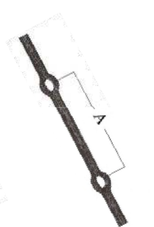
08.023 H 2000 mm A 140 mm ∅ 14 mm 14 otworów ∅ 14mm 2,420 kg
