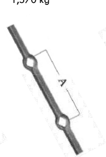
08.123 H 2000 mm A 125 mm ◇ 14x14 mm 15 otworów ◇ 14mm 3,080 kg
