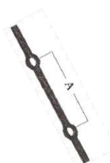
08.115 H 2000 mm A 125 mm ∅ 14 mm 15 otworów ∅ 14mm 2,420 kg
