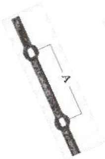
08.001 H 2000 mm A 140 mm □ 14x14 mm 14 otworów □ 14mm 3,080 kg
