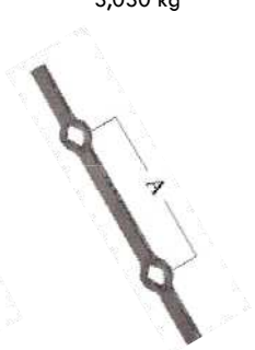
08.127 H 2000 mm A 125 mm □ 14x14 mm 14 otworów ◇ 14mm 3,080 kg
