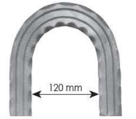
12.036 H 200 x L 200mm || 40x6 mm 0,950 kg
