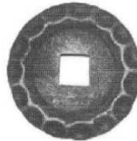
13.318.16 Ø 75 mm □ 16,5 mm gr. 5 mm 0,140 kg
