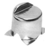
STOPER DO BRAMY SKRZYDŁOWEJ H 103 x L 103 mm 0,375 kg
