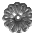
14.010 Ø 68 mm gr. 1,5 mm 0,030 kg
