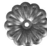
14.011 Ø 97 mm gr. 1,5 mm 0,085 kg
