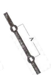
08.119 H 2000 mm A 125 mm □ 14x14 mm 15 otworów □ 14mm 3,080 kg
