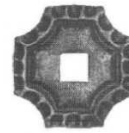
13.316.16 H 75 x L 75 mm □ 16,5 mm gr. 5 mm 0,160 kg
